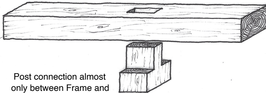
Ständer und Riegel Verbindung in Dijari
