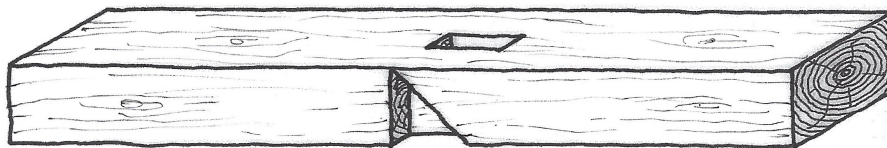
Tür und Fenstereckverbindung in Satkhol Zwischen 1900 und 1930 gebaut
